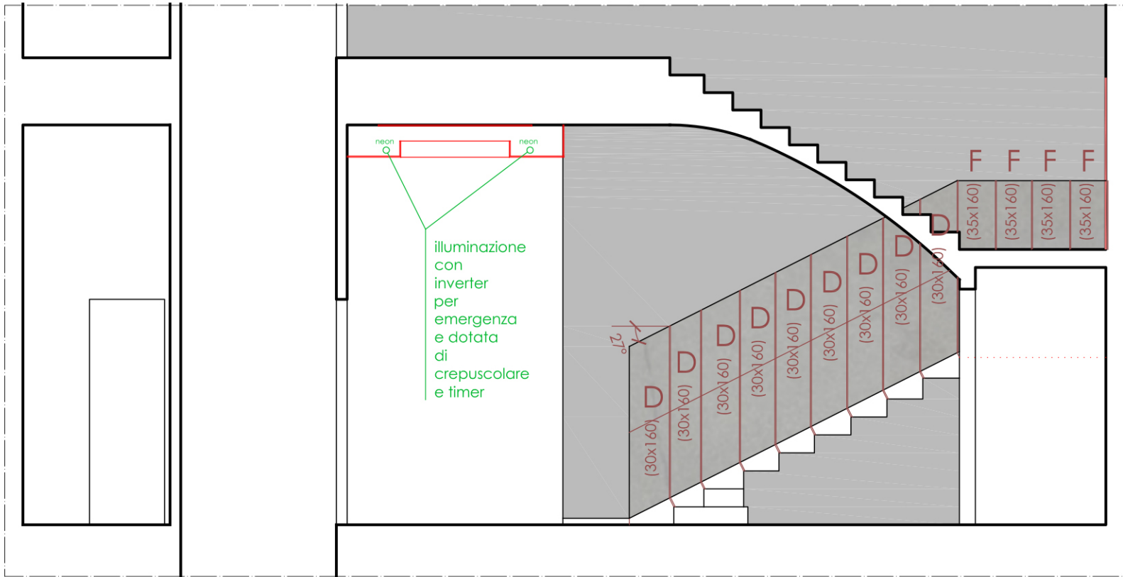
SEZIONE B-B'
